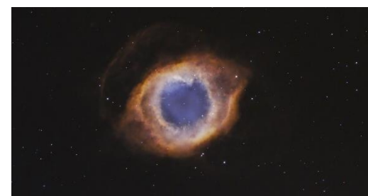
Isten szeme Hélix-köd
